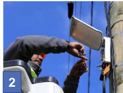
La fibre est en attente dans le PBO au niveau d'un poteau de votre rue
